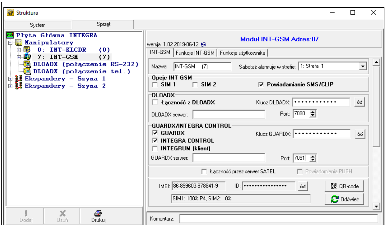
Rys. 9. Program DLOADX: ustawienia modułu INT-GSM podłączonego bezpośrednio do centrali INTEGRA / INTEGRA Plus.
